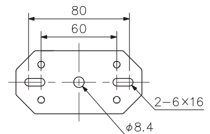
スピーカー取付部拡大図 (縮尺: 1/3)
